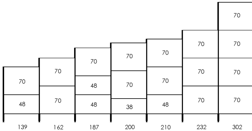
Perusjärjestelmä, jalka H19
